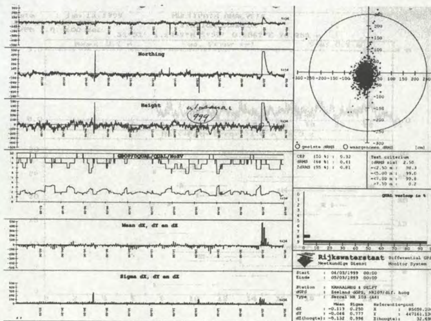
Figuur 14 Digmosy: coördinaat, kwaliteit en statistische informatie .
