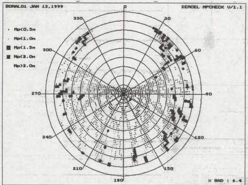
Figuur 13 Mpcheck: multipad skyplot.
