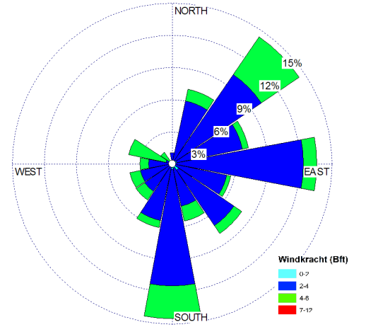
Marollegat gem windsnelheid 9 februari t/m 9 maart 2011
