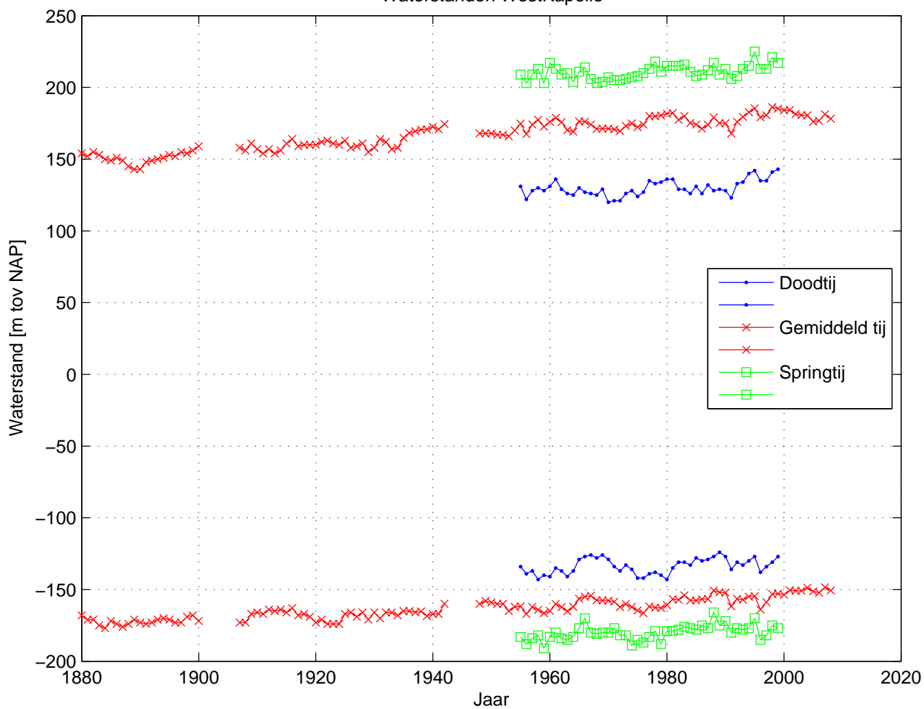
Waterstanden WestKapelle
