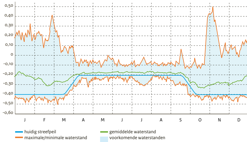
Figuur q: Waterstanden in het IJsselmeer in de periode 1976 t/m 2012.
