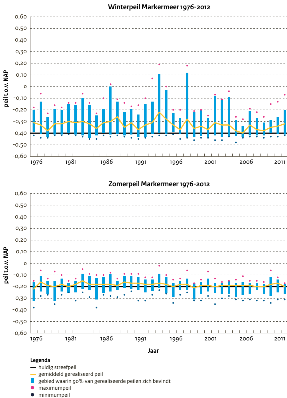
Figuur 10: Streefpeilen en gemeten waterstanden in het Markermeer.
