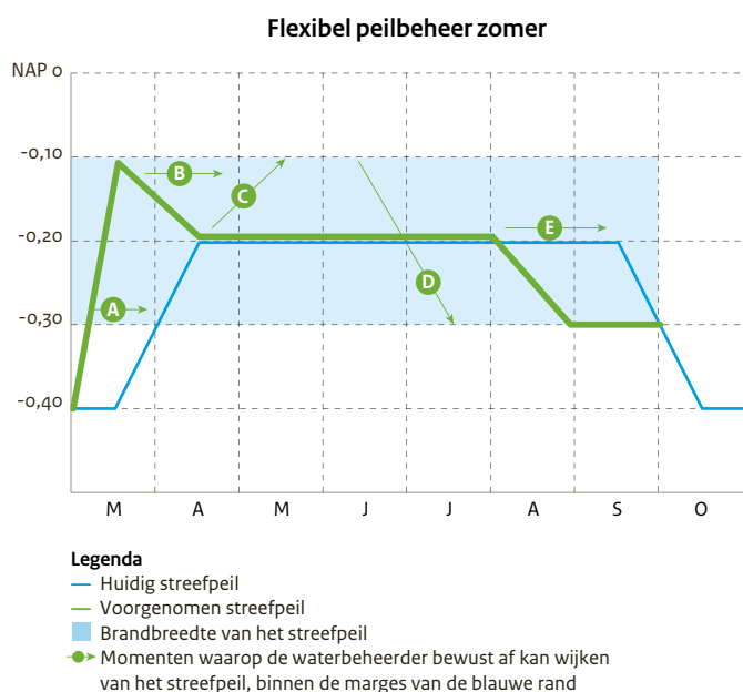
Figuur 6: Voorgenomen en huidig zomerstreefpeil in IJsselmeer en Markermeer.
