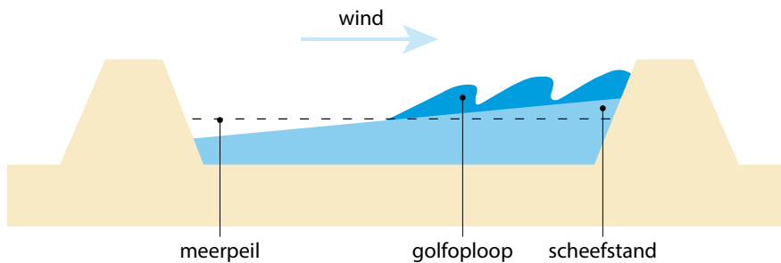
Figuur 3: Effect van golfoploop en scheefstand op de waterstand.
