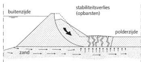
Figure 2.10 Uplift (opdrijven) vs rupture (opbarsten), source: TAW (2001).
