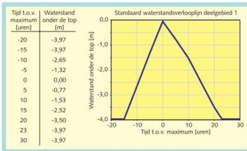
Figuur 7.8 Voorbeeld standaard waterstandsverlooptij [Min V en W, 2007]
