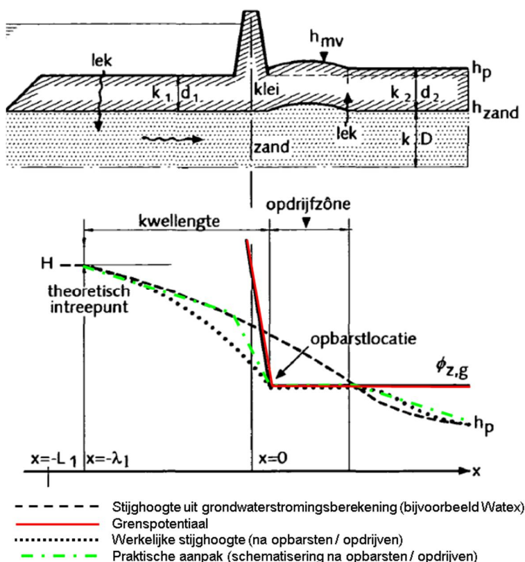
Figuur C.2 Dijk met voorland en ondergrond; Stijghoogte in zandlaag, grenspotentialiaal en opdrijfzone
