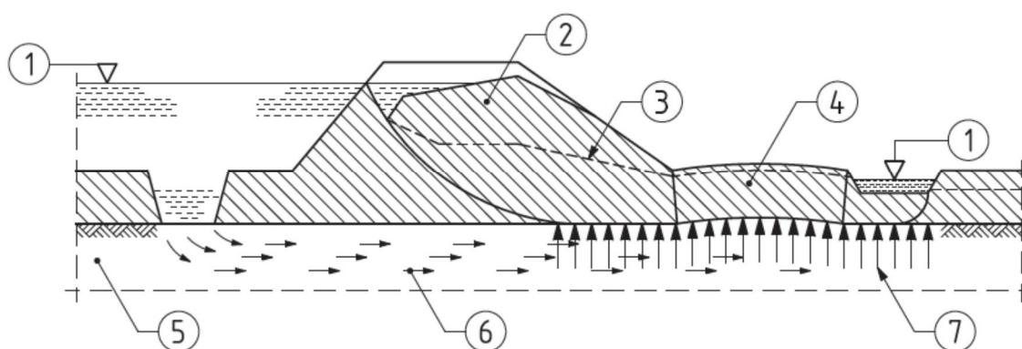
Figuur C.4 Principe van het rekenmodel Lift-Van voor opdrijven [zie Eurocode 7 ref.7] met 1 Vrij waterniveau, 2 Dijklichaam, 3 Waterstand in de dijk, 4 Grondmoot, die horizontaal en door de opwaartse waterdruk wordt belast ("drukstaaf"), 5 Diepe zandlaag, 6 Grondwaterstroming en 7 Opwaartse waterdruk onder de deklaag
