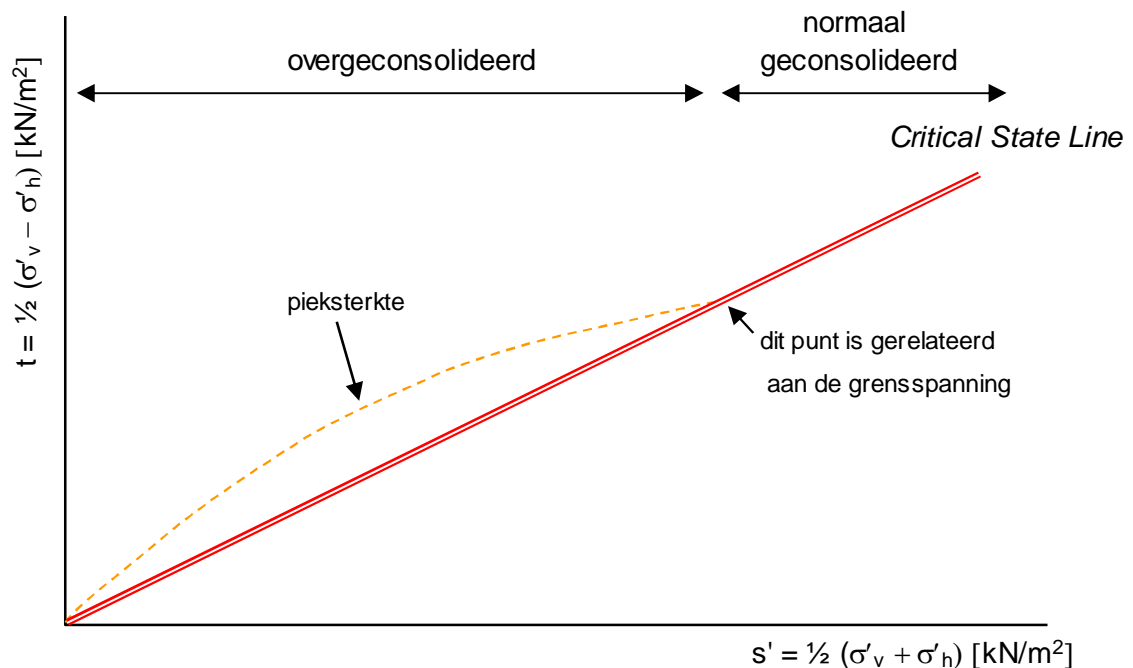
Figuur C.5 Karakterisering van de schuifsterkte volgens het Critical State Soil Mechanics raamwerk (CSSM)
