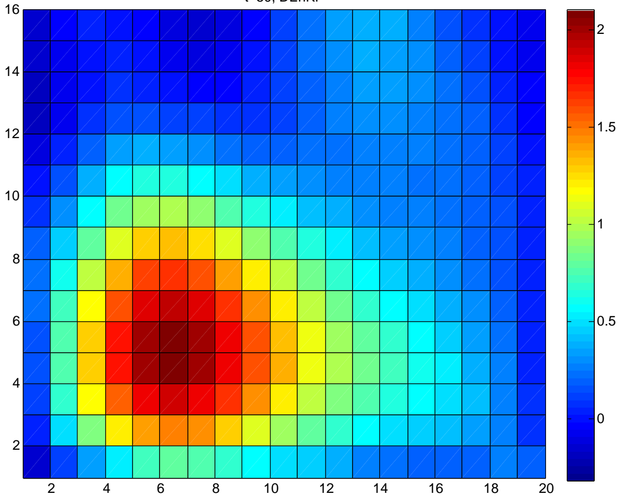
t=50, DEnKF
